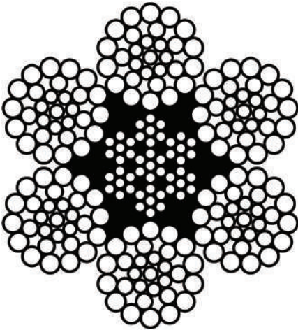
6x36 IWRC • Fatigue resistant • Abrasion resistant
